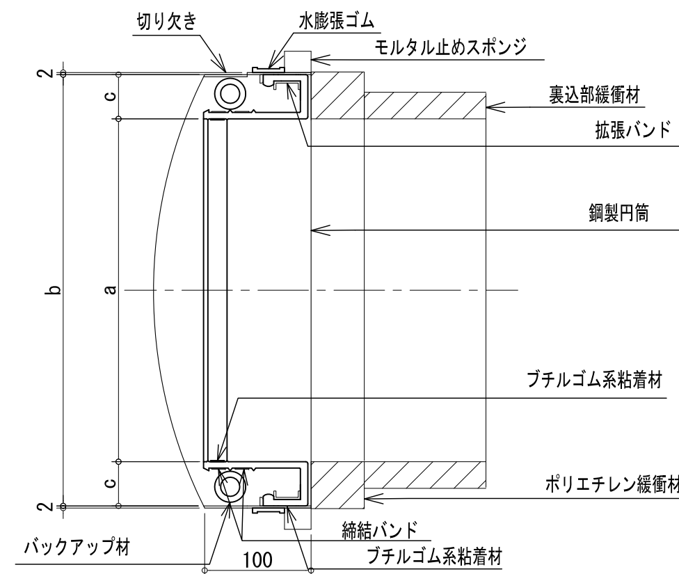
A-A断面図
